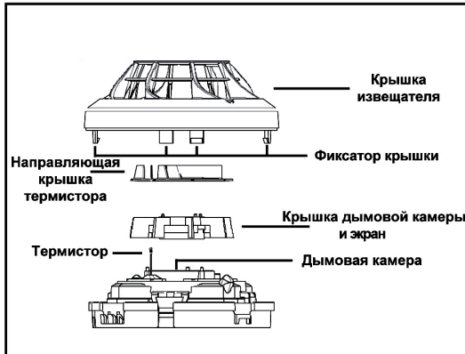
Рис.2: Обслуживание извещателя
