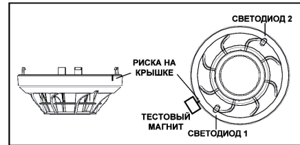
Рис. 3: Тестирование магнитом
