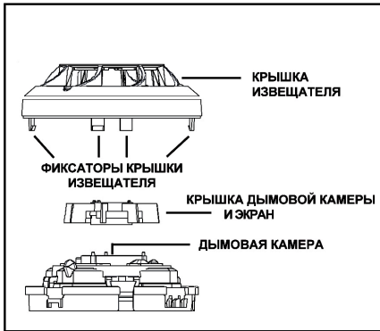
Рис.2: Обслуживание извещателя
